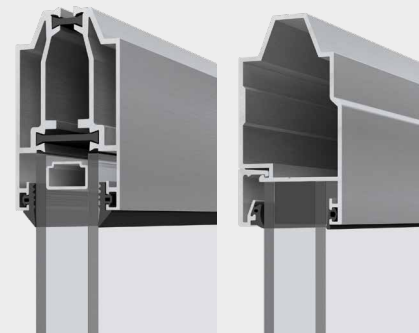
ПАНОРАМНАЯ ПАНЕЛЬ ИЗ ПРОФИЛЕЙ С ТЕРМОРАЗДЕЛЕНИЕМ T-BRIDGE
